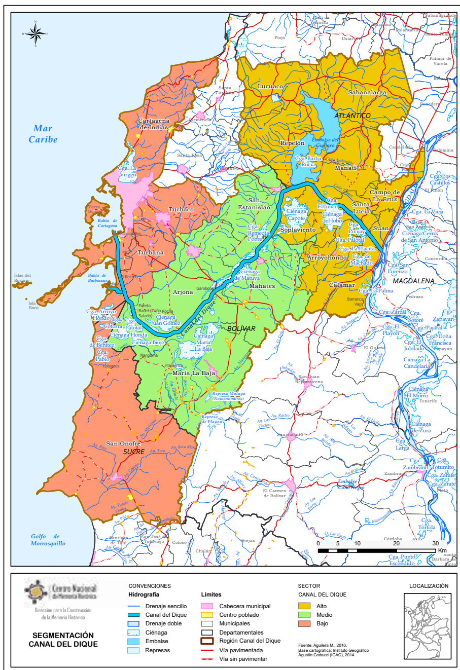
Figura 2. Segmentación del Canal del Dique.
