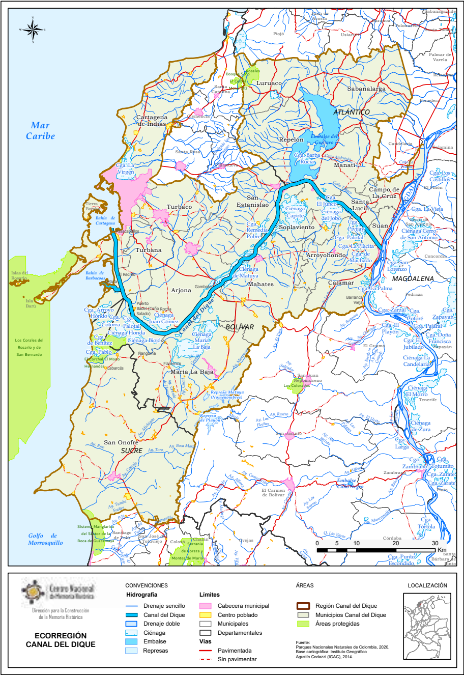
Figura 1. Ecorregión del Canal del Dique. Fuente: elaborado por el CNMH con información del Consorcio Dique (2016a).
